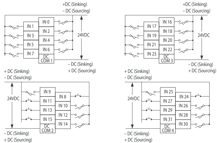
1769-IQ32
