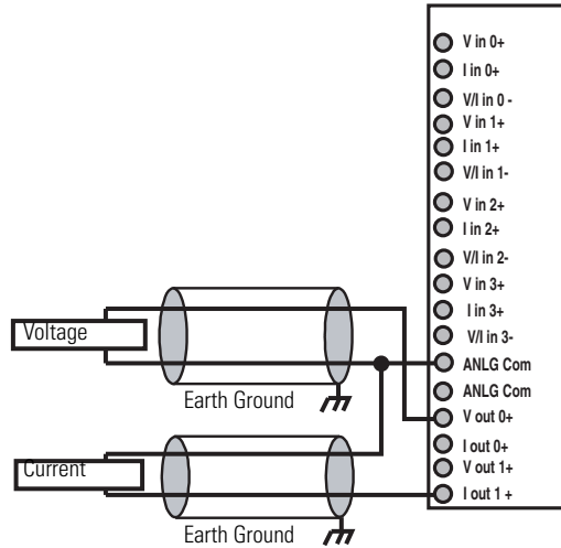
1769-IF4FXOF2F Outputs
