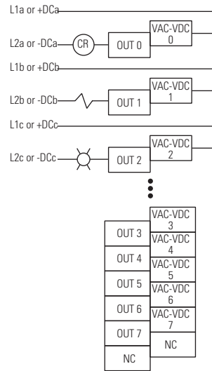
1769-OW8I
